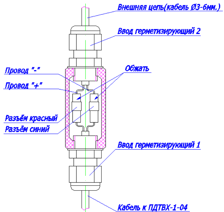
Рис. 2 Узел соединительный
